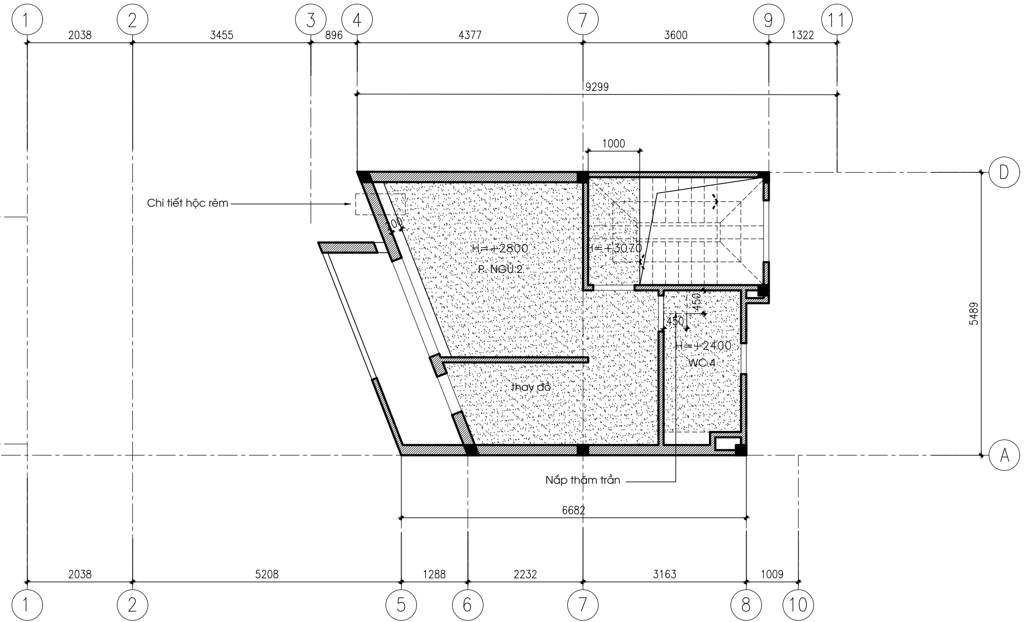
MẶT BẰNG TRẦN THẠCH CAO LẦU 2
