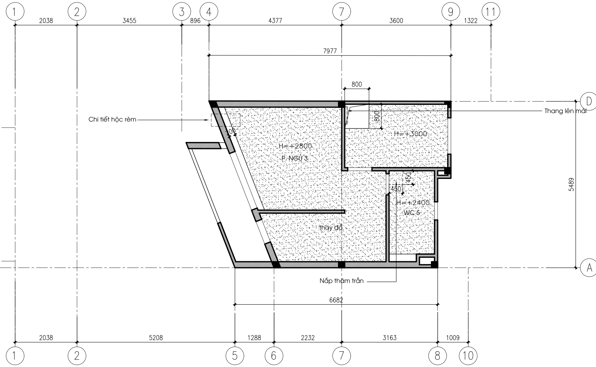
MẶT BẰNG TRẦN THẠCH CAO LẦU 3
