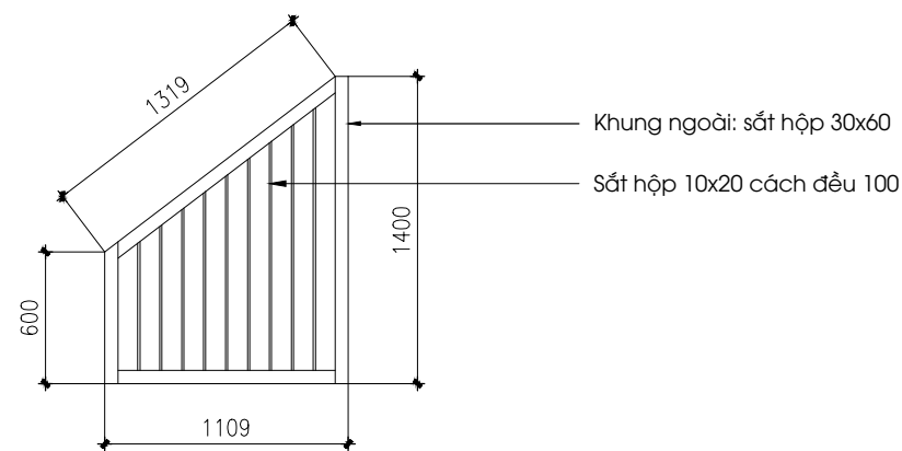
MẶT ĐỨNG BÊN
