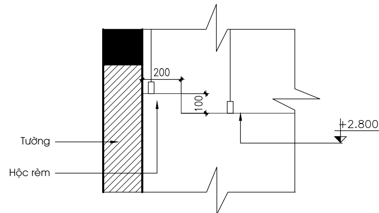
CHI TIẾT HỘC RÈM
