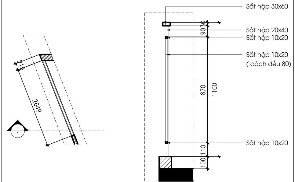
MẶT BẰNG
