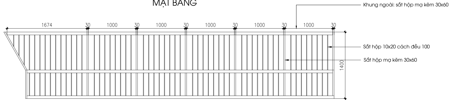
MẶT ĐỨNG
